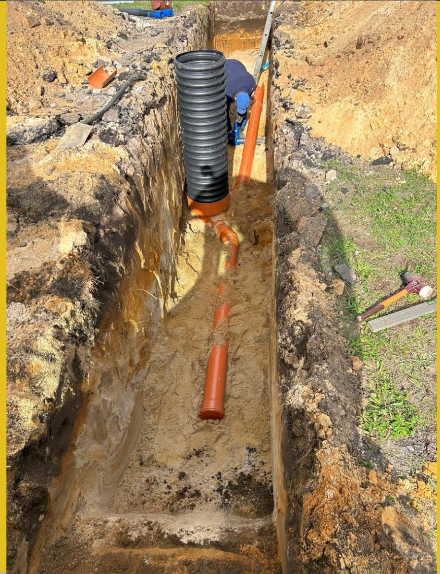
Budowa kanalizacji ul. Bukowa
