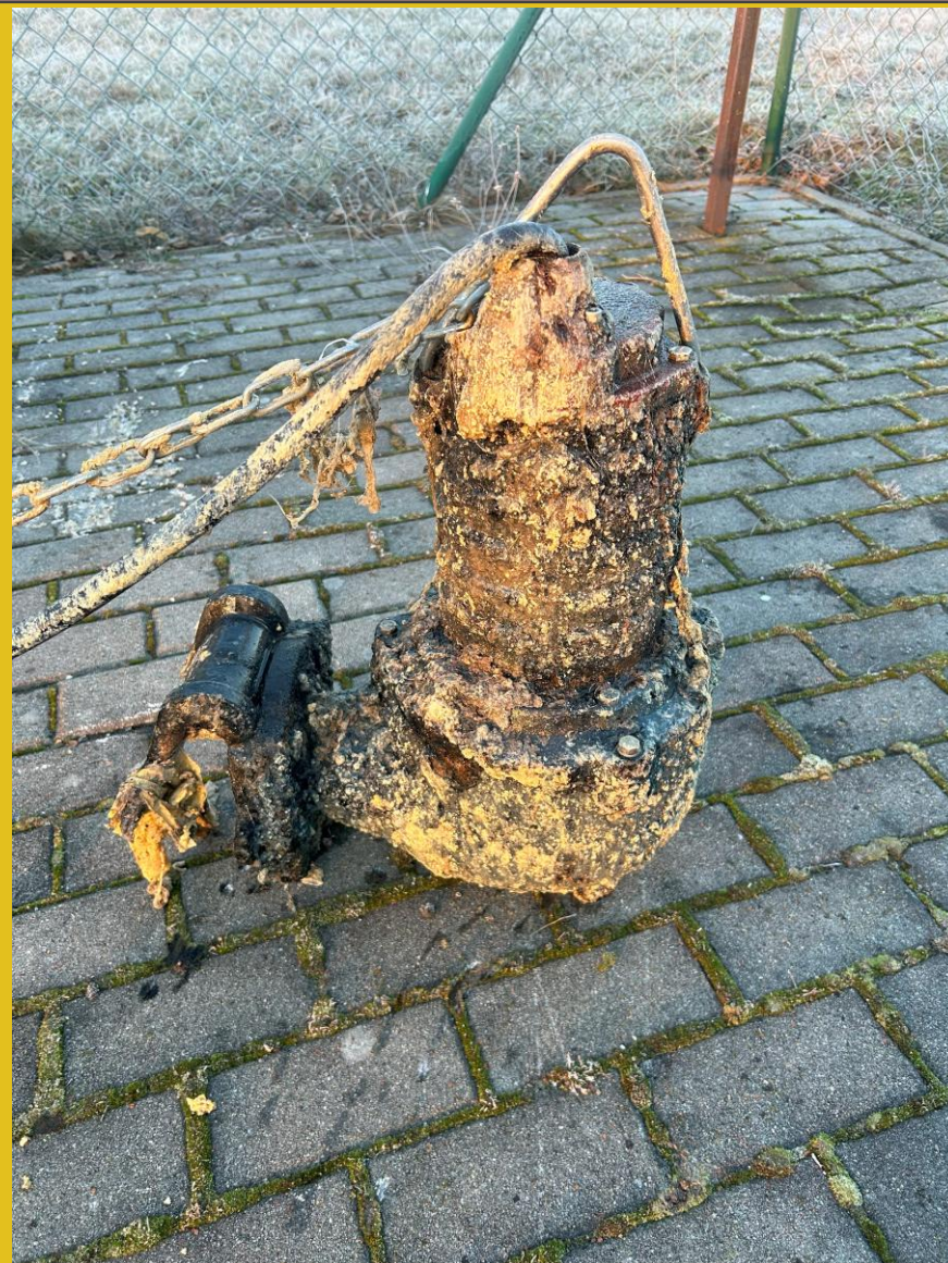
Zniszczenia w przepompowniach
