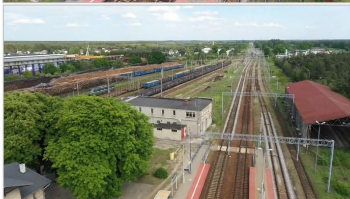
Widok w kierunku wschodnim (linia do Lublińca i Zawadzkiego). Po prawej hala przegladów.
